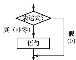
图1 if 语句流程 1
