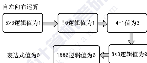
【图】 5>3\&\&8<4-!0 的计算过程
