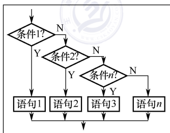
图3 多分支语句
